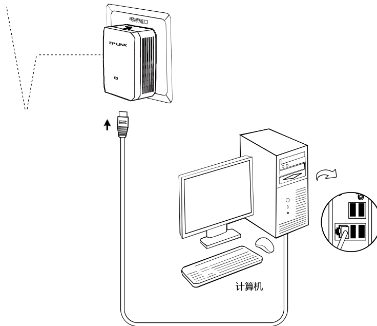
图2-3 终端连接图
