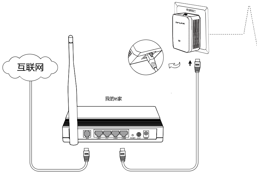
图2-2 网络连接图
